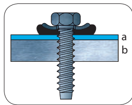
Łącznik dokręcony zbyt dużym momentem. Efekt: brak szczelności połączenia, ograniczona nośność połączenia.
